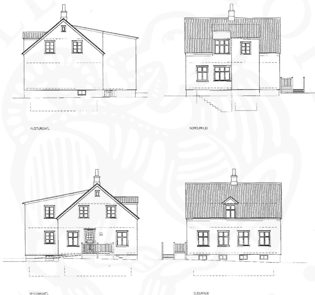
Mynd 8: Samþykktar teikningar af Ráðagerði frá 1997. Teiknistofan Skólavörðustíg 28/ Stefán Örn Stefánsson og Grétar Markússon
