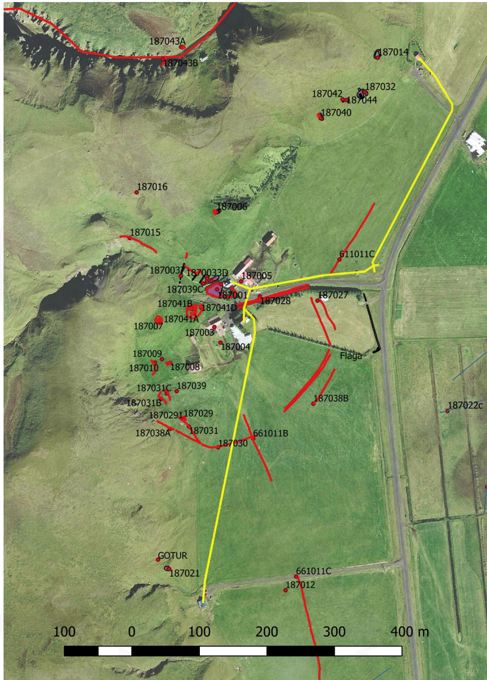
Fyrirhuguð lega ljósleiðara að íbúðarhúsum í landi Flögu. Loftmynd: Loftmyndir ehf.
