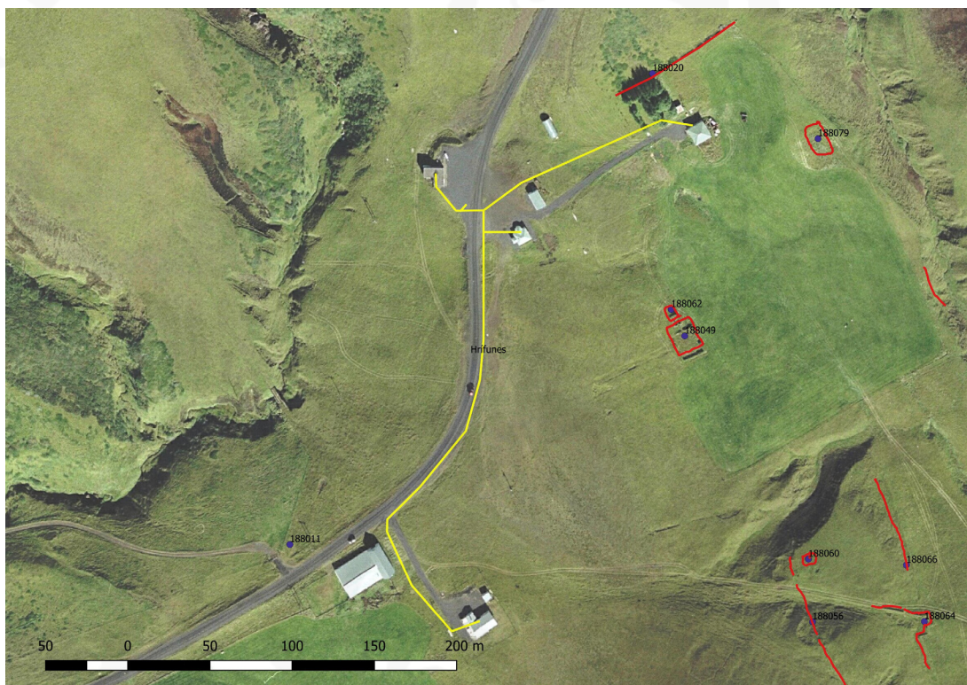
Fyrirhuguð lega ljósleiðara að íbúðarhúsum í landi Hrífuness. Loftmynd: Loftmyndir ehf
