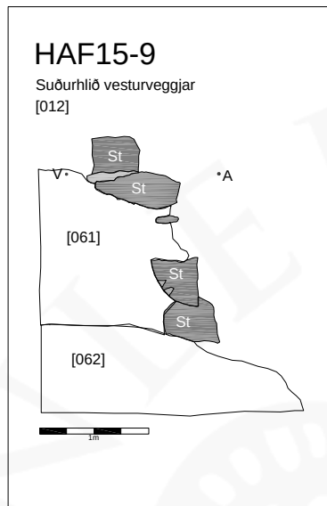
Teikning 7: Suðurhlið vesturveggjar.
