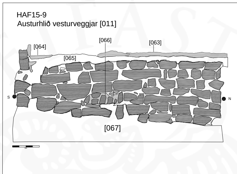
Teikning 4: Vesturveggur
