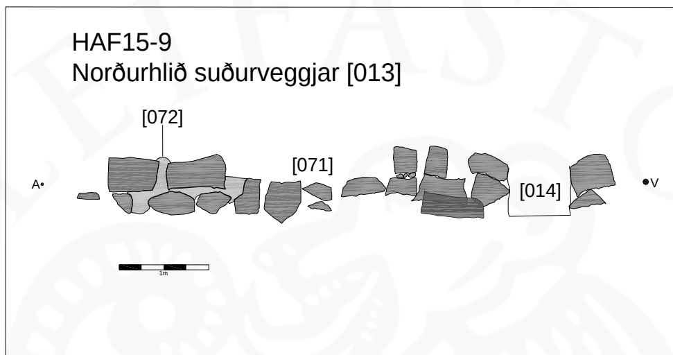
Teikning 6: Suðurveggur
