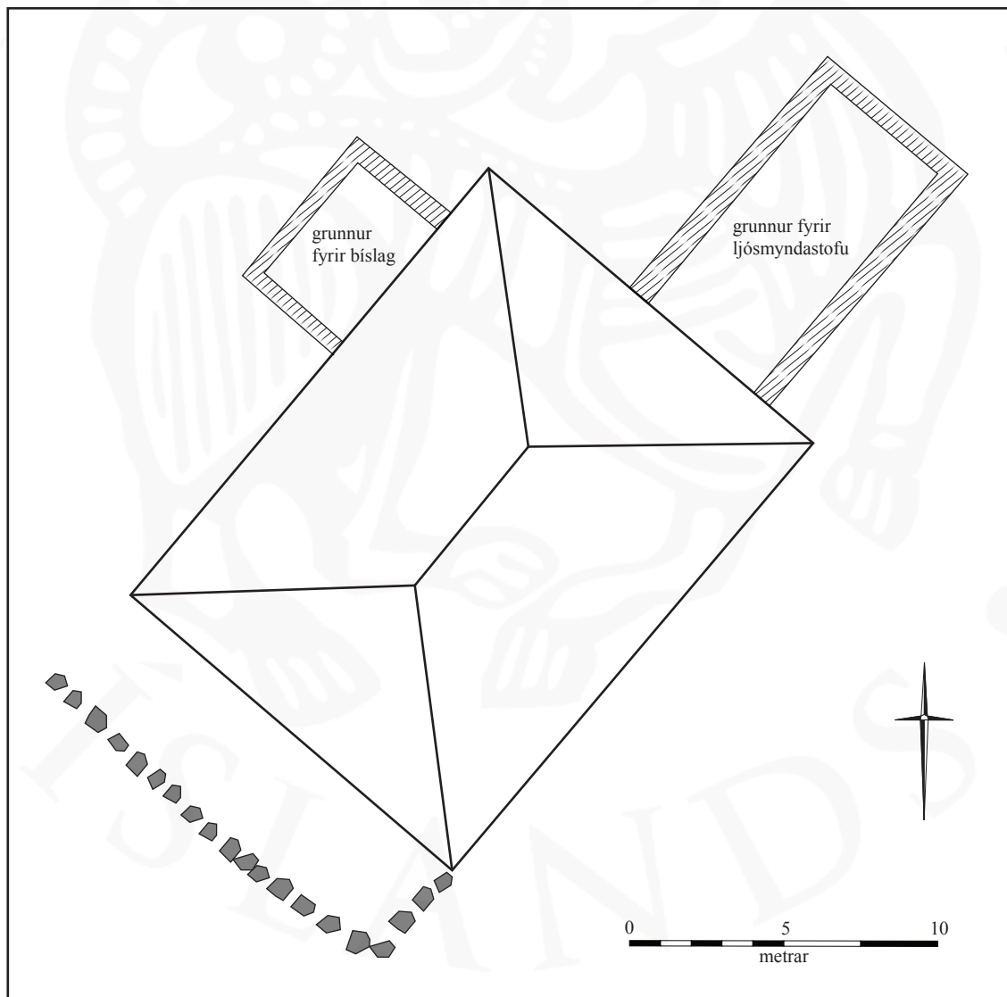
Uppdráttur af timburhúsi 002
