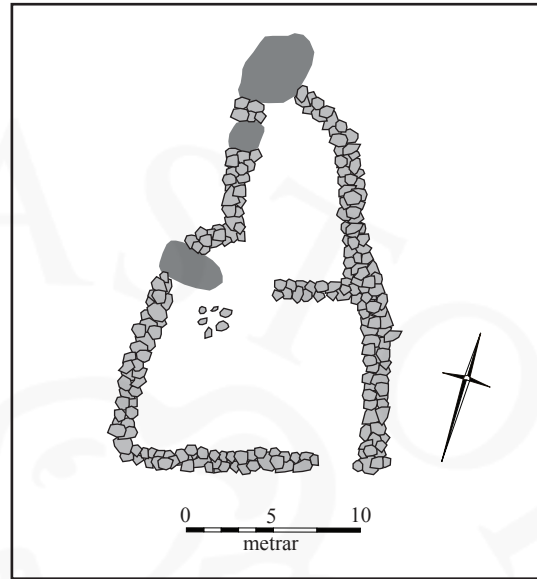
Uppdráttur af rétt 012
