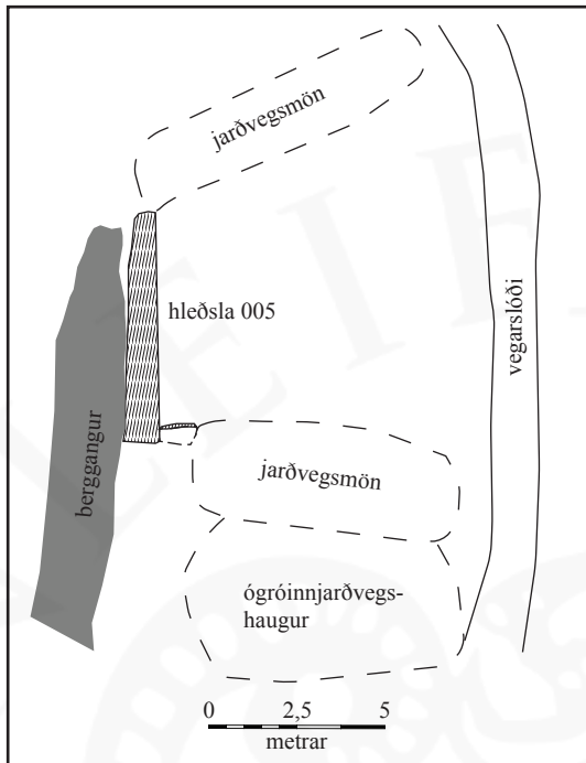
Uppdrátturinn sýnir 13m grjóthlaðinn sem eru einu leifar fjárhúss 005
