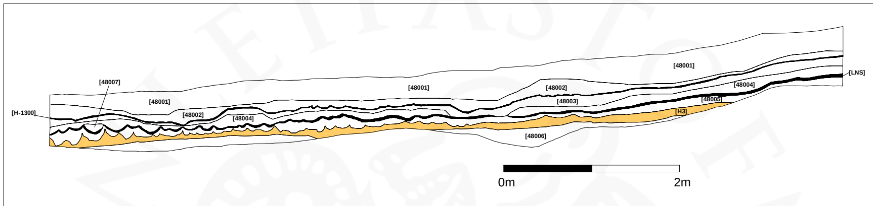
Mynd 7: Teikning af norðursniði könnunarskurðar SK-312048. Lögnum sem sjást á teikningunni er lýst í töflu 4.
