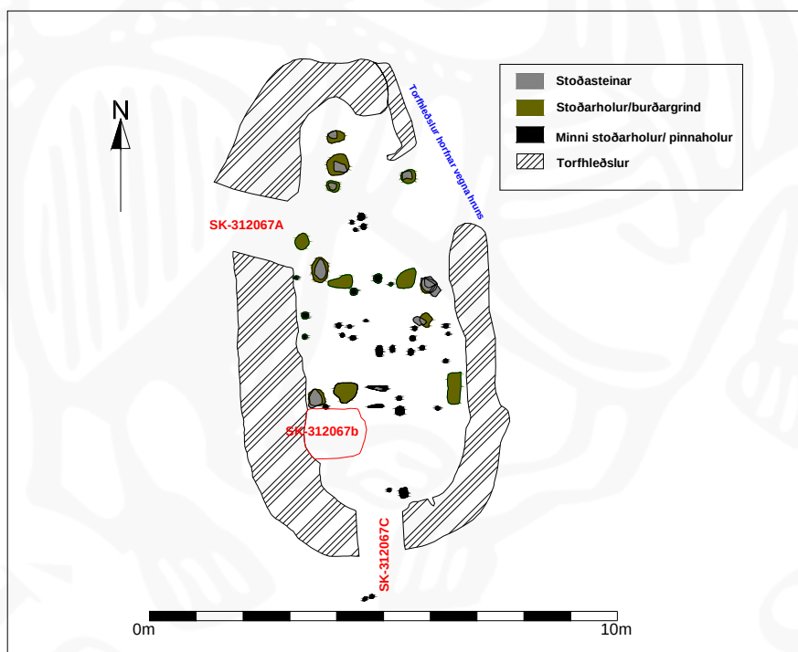
Mynd 29: Einfölduð teikning af tóft SP-312:067 með stoðarholum og stoðarsteinum
