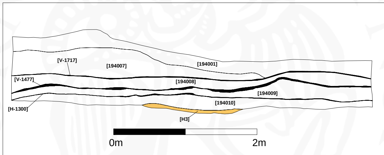
Mynd 15: Teikning af vestursniði könnunarskurðar SK-313194B.
