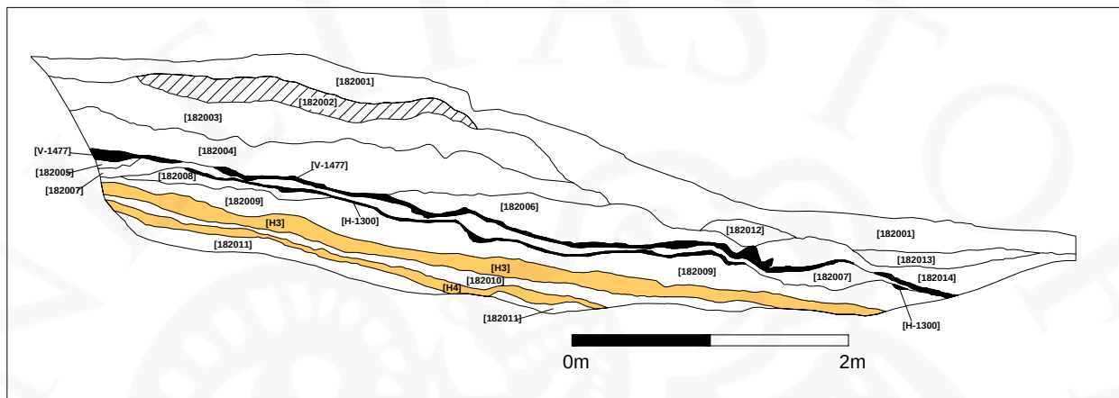
Mynd 18: Teikning af suðursniði könnunarskurðar SK-313182A.
