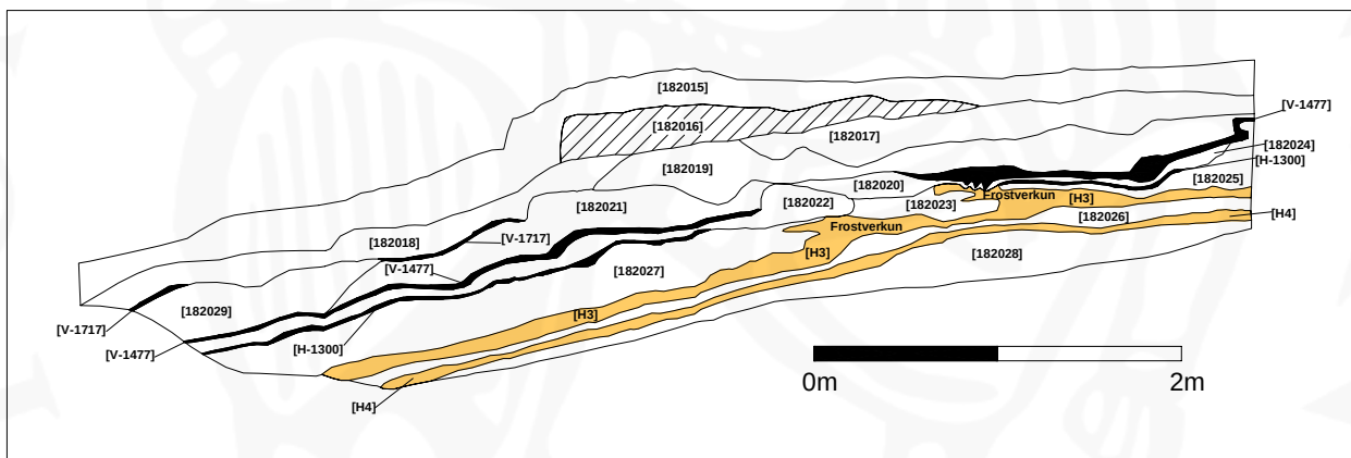
Mynd 19: Teikning af norðursniði könnunarskurðar SK-313182B.
