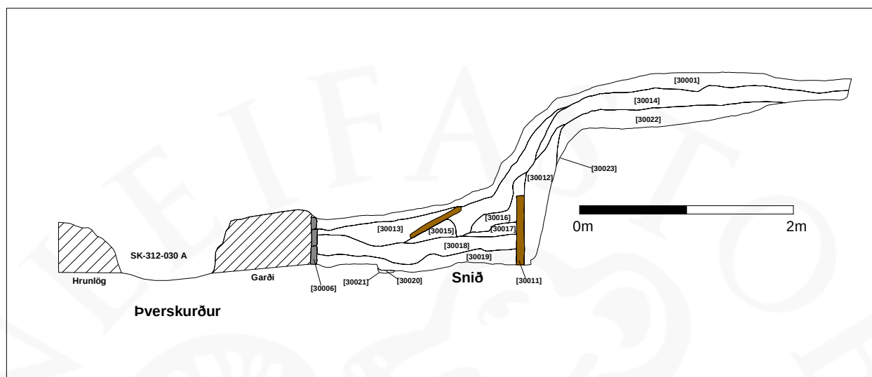
Mynd 13: Teikning af austursniði könnunarskurðar SK-312030B ásamt þverskurði yfir garðann í fjárhúsinu og könnunarskurð SK-312030A. Má m.a leifar timburpilsins upp að suðurvegg fjárhússins.
