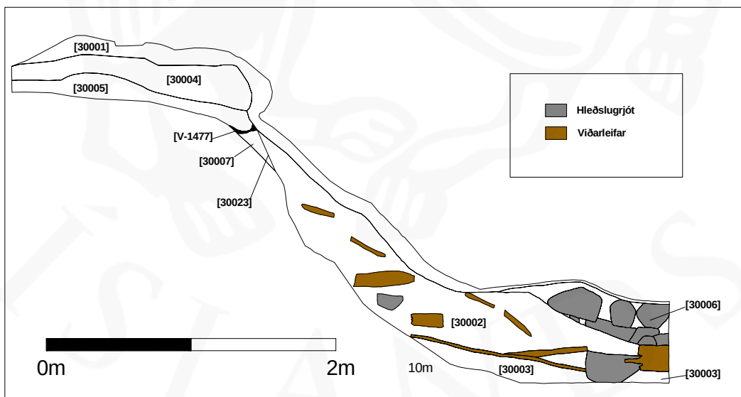
Mynd 12: Teikning af suðursniði könnunarskurðar SK-312030A, þar sem m.a má sjá leifar timbers úr þiljum og stoðgrind fjárhússins ásamt grjóthleðslum í garða. Er lögum sem sáust í sniðinu lýst nánar í töflu 5 hér að neðan.
