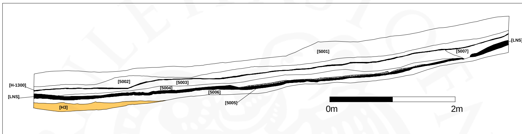
Mynd 6: Teikning af norðursniði könnunarskurðar SK-312005. Lögnum sem sjást á teikningunni er lýst í töflu 3.
