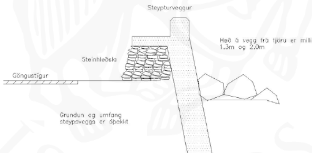
Mynd 1: Suðursnið í gegnum garðinn sem sýnir gerð hans. Fengin úr útboðsgögnum
