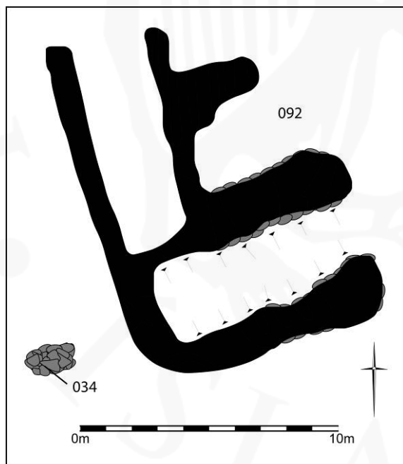
Uppdráttur af nausti 092
