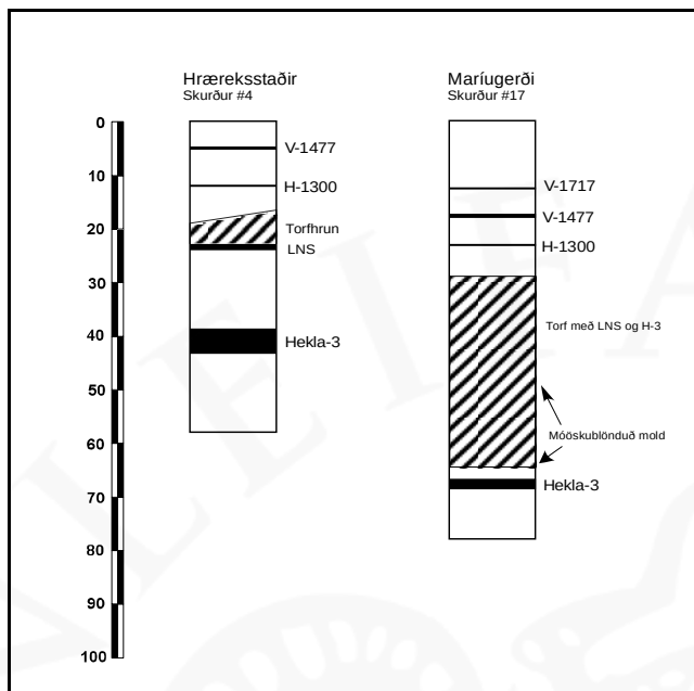
Mynd 1. Jarðvegssnið frá Hræksstöðum og Maríugerði, Kelduhverfi.
