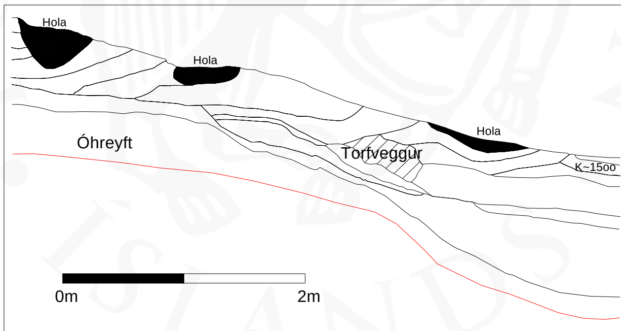
Mynd 40: Einfölduð mynd af hluta suðursniðs SK18 þar sem sjá mátti slitrur af torfvegg
