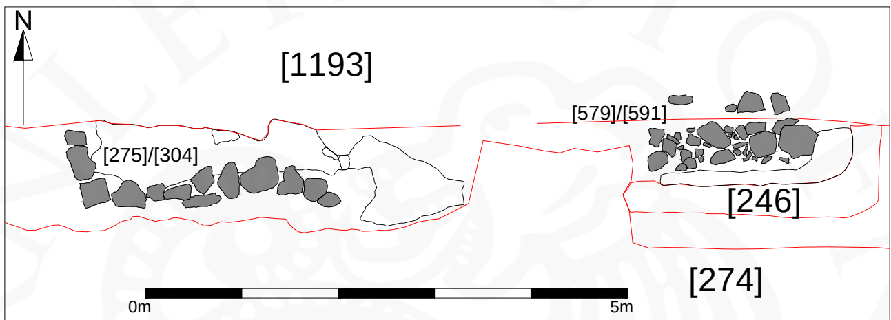
Mynd 9: Teikning af veggjarbrotum [275]/[304] og [579]/[591]
