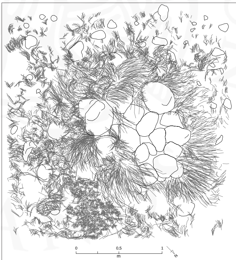
Mynd 13. Varða í Sauðárdal. Flatarteikning þegar helmingur vörðunnar hafði verið fjarlægður. (Mynd Fornleifastofnun Íslands, GG.)
