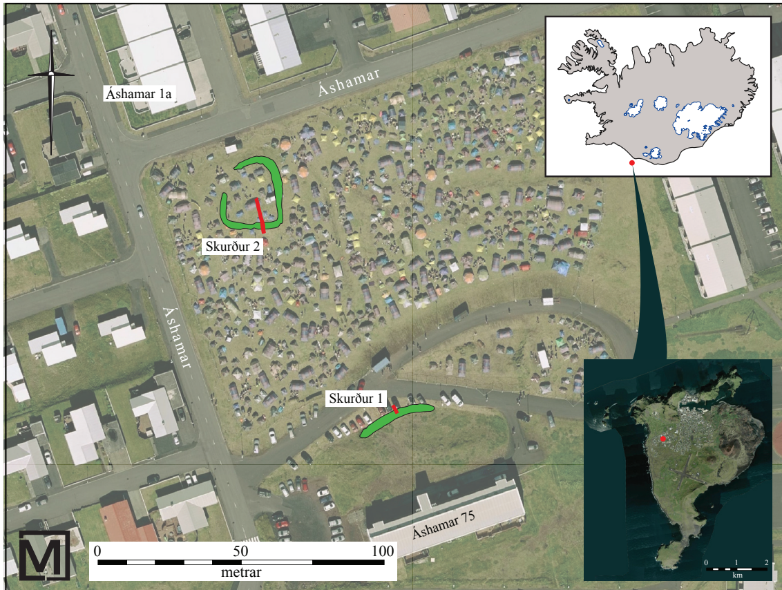
Myndi 1. Loftmyndin sýnir staðsetningu rannsóknarsvæðis með rauðum punkti. Yfir loftmyndina hefur verið varpað uppmælingum frá Minjastofnun Íslands og eru þær sýndar með grænum fláka (uppmæling fengin hjá Minjastofnun Íslands). Uppmælingum af rannsóknarskurðum hefur einnig verið varpað yfir loftmyndina og eru þeir sýndir með rauðum fláka. Loftmynd: Loftmyndir ehf.
