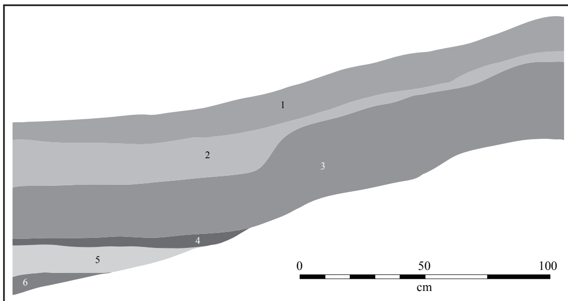
Mynd 7. Snið í skurði 2 sem grafinn var í tóft af gerði um 30m sunnan við Áshamar nr. 1a. Engar fornleifar sáust í sniðinu. 1, grasrót - yfirborð. 2, Vikur frá Vestmannaeyjargösinu 1973 (aðfluttur). 3, Dökkbrúnn jarðvegur. 4, Forsöguleg gjóska úr Kötlu. 5, Ljósbrúnn jarðvegur. 6, Forsöguleg gjóska úr Kötlu. Sniðið var teiknað í austurhlíð skurðar.
