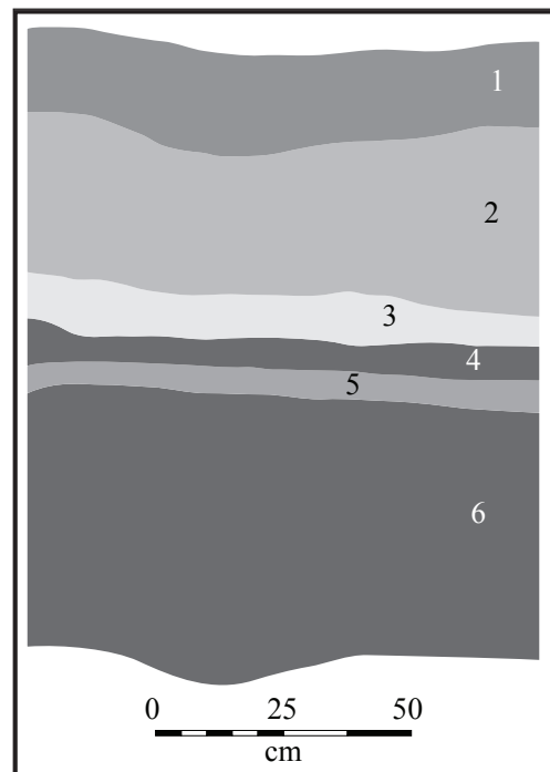
Mynd 4. Snið í skurði 1 sem grafinn var í garðlag 30m norðan við Áshamar nr. 75. Engar fornleifar sáust í sniðinu. 1, grasrót - yfirborð. 2, Uppmokaður sandhryggur. 3, Brúnleitur jarðvegur. 4, Vikur frá Vestmannaeyjargösinu 1973 (aðfluttur). 5, Brúnleitur jarðvegur. 6, Vikur frá Vestmannaeyjargösinu 1973 (aðfluttur). Sniðið var teiknað í norðurhlið skurðar.
