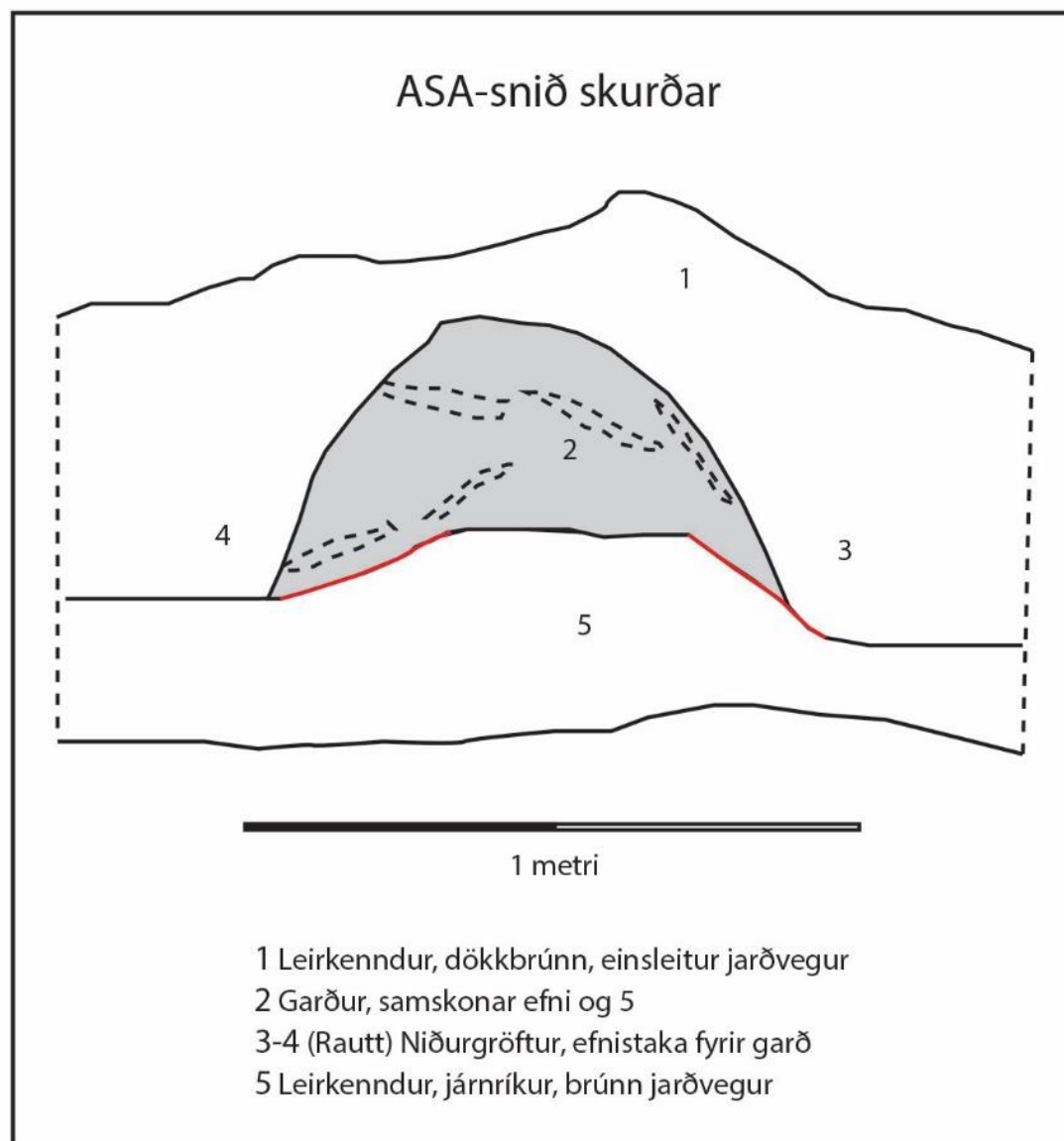
Mynd 2 Sniðteikning, horft til ASA
