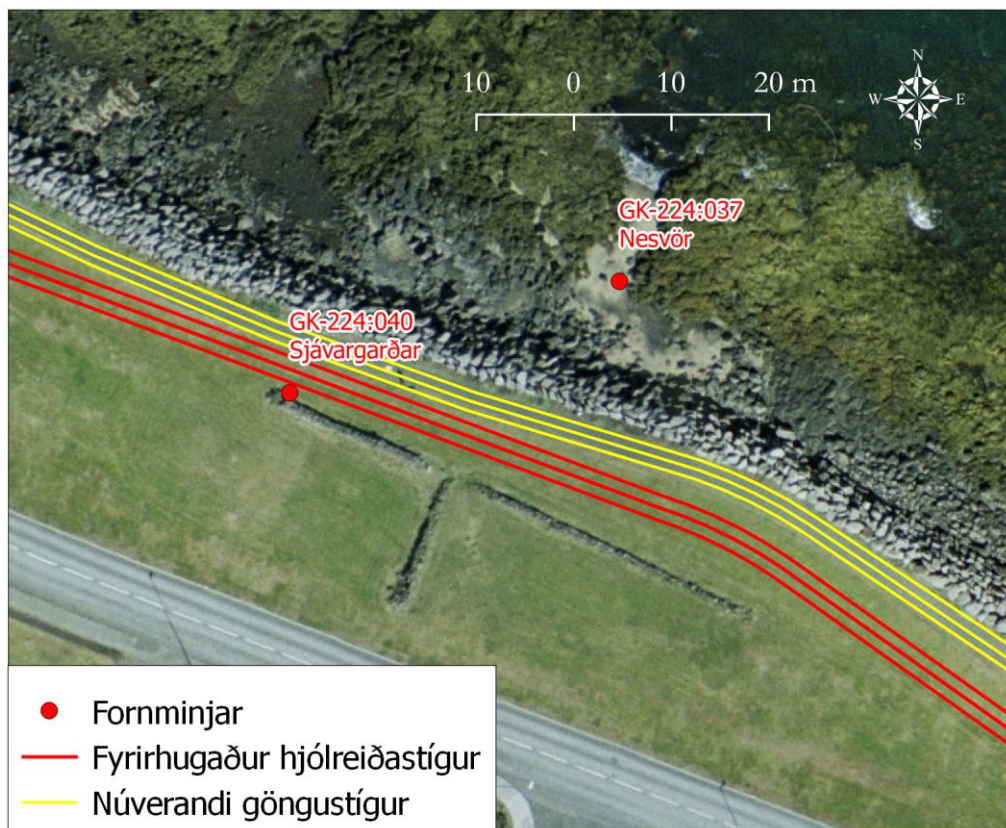
Mynd 4: Sjavargarðar
