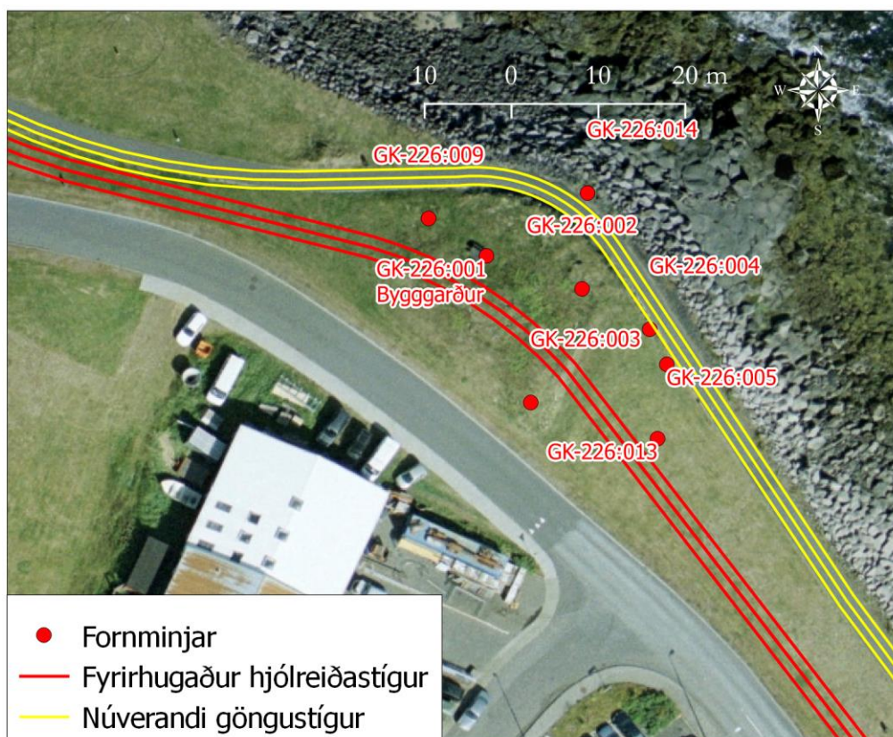
Mynd 5: Bygggarður
