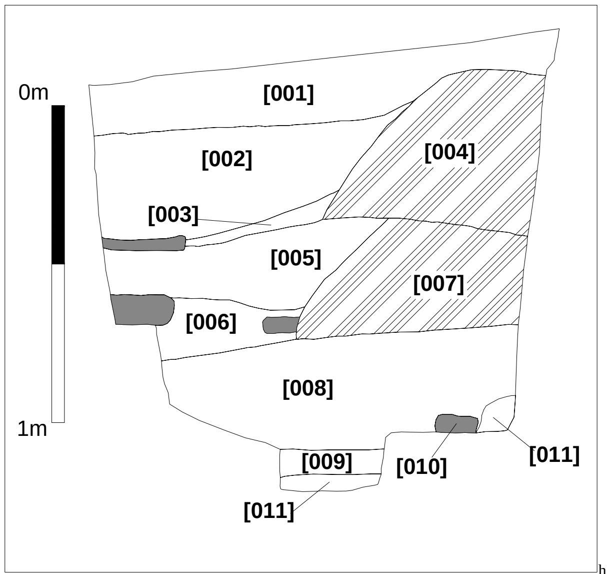
Mynd 22. Austursnið í skurði í tóft í Skógarnesi.
