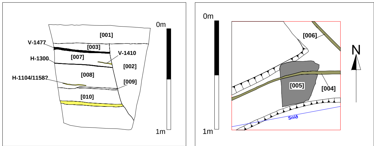
Mynd 4-5. Skurður A. Suðursnið t.v. og grunnmynd t.h. Gula linsan er H3
