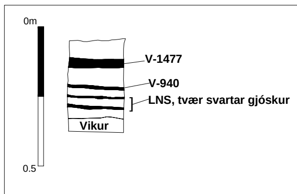
Mynd 11. Einfaldað snið í skurði A. Öll lögin eru óhreyfð.
