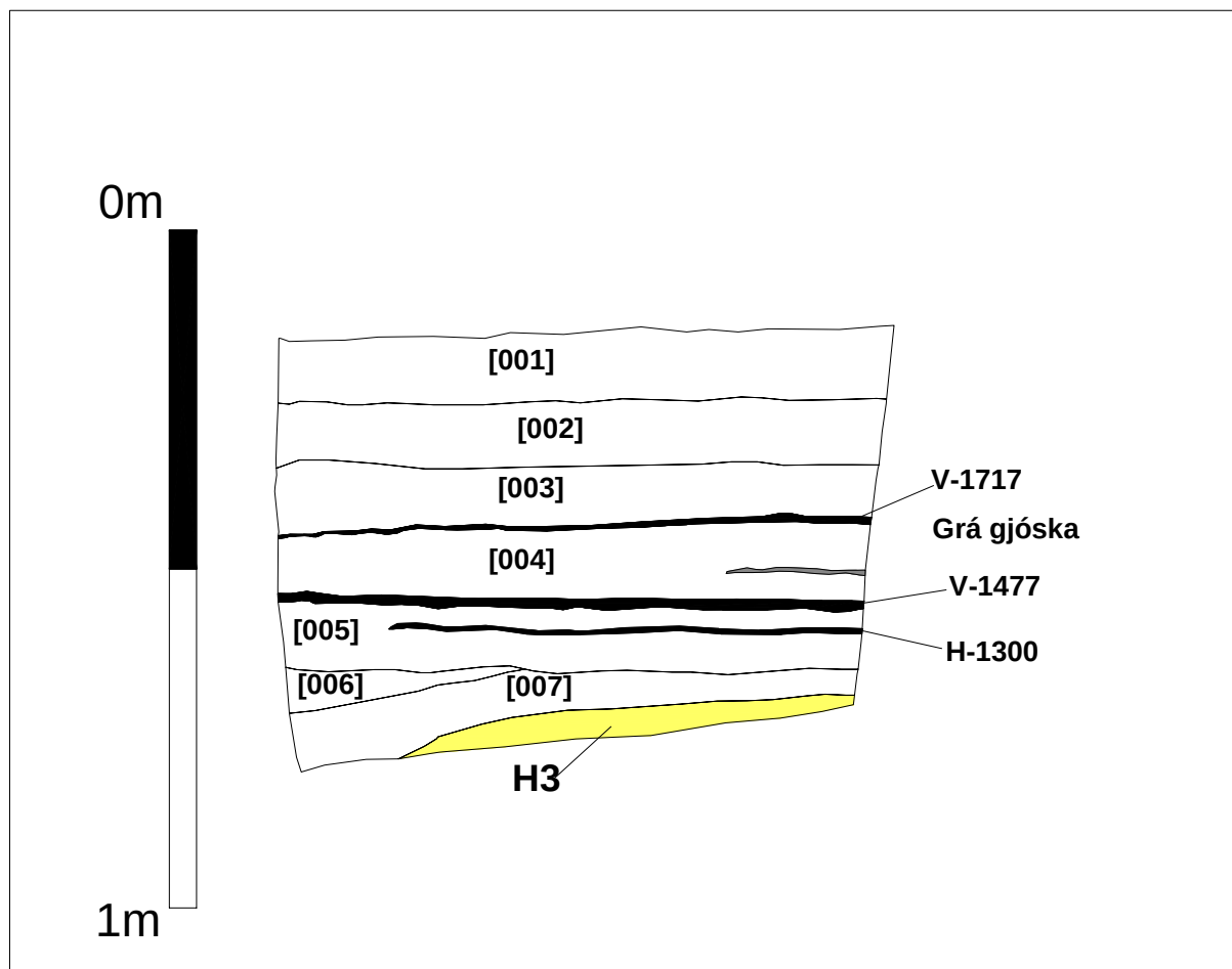
Mynd 6. Skurður B, suðursnið.
