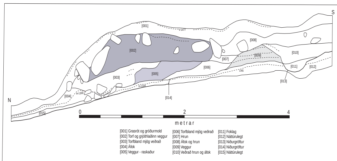
Sniðteikning garðsins í landi Hamars
