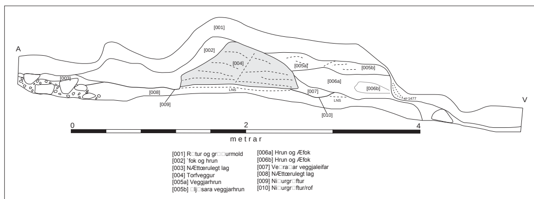
Snið í Skessugarð í landi Tungufells
