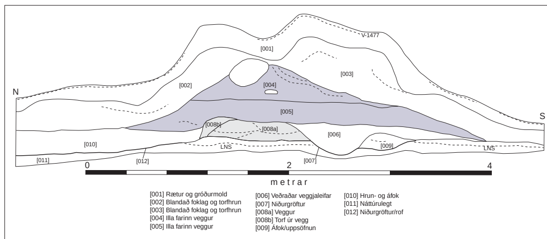
Snið Þvergarðs, frekari útlistanir á mannvistarlögum sniða er að finna í viðhengi 2
