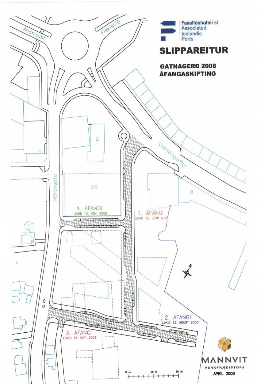
Mynd 1: Skipulagsuppráttur, frá verkfræðistofunni Mannvit, sem sýnir áhrifasvæði framkvæmda neðan Mýragötu og áfangaskiptingu þeirra.
