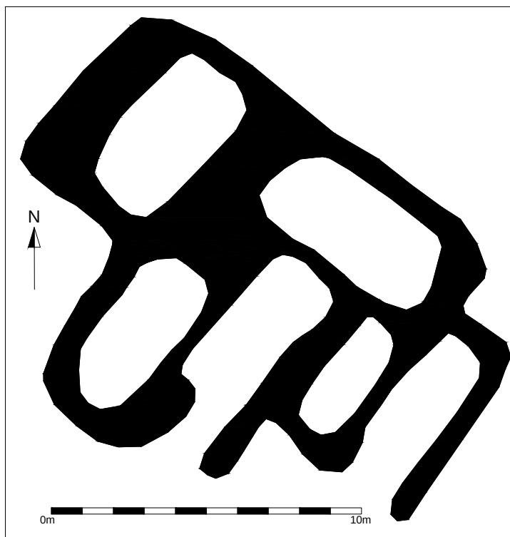
Teikning 31: Tóft NP-062:061 í Vellankötlu. Sjá einnig teikningu 12 hér frammar
