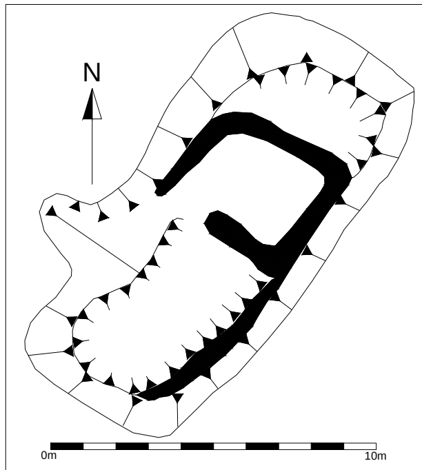
Teikning 38: Tóft NP-062:070 á Selibrekkuhólum.
