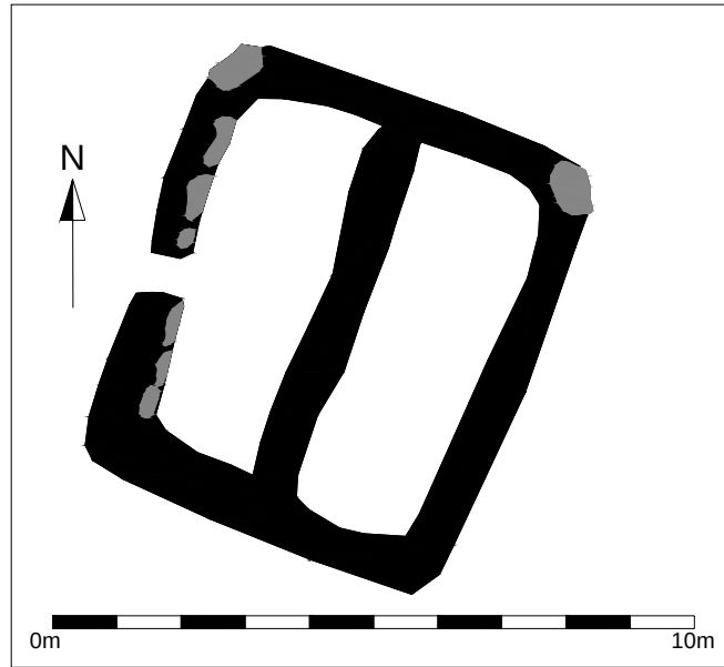
Teikning 19. Hrútakofatóft NP-062:042
