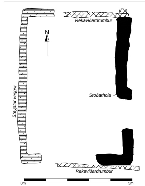
Teikning 4: Kofahólstótt, NP-062:007
