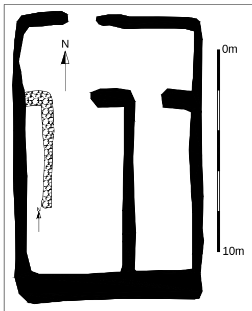
Teikning 10: Hesthústóft NP-062:016.
