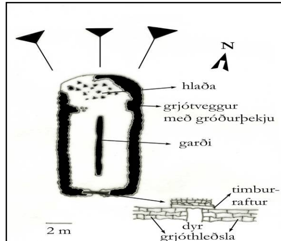
Teikning 3: Beitarhús. SF-188:015
