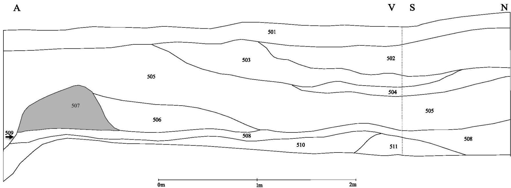
Mynd 14. Skurður 5, sniðteikning af völdum hluta suðursniðs og vestursniðs. Garðlagið er grálitað. Brotalínan sýnir SV horn skurðar.
