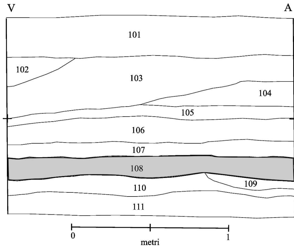
Mynd 4. Skurður 1, sniðteikning norðursniðs.
